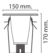
WL-L4015-3YY 130 W150xH170mm E27=1x40W ອລຸມິນຽມ
