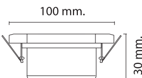
WL-DX012CH-SL 240 W100xH30 mm MR16=1x50W ไม่ร้อนหลอด
