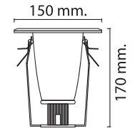
WL-P4016-2SS 130 W150xH170mm E27=1x40W ឧត្តមជ័យ
