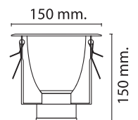
WL4032-A-KG 180 W150xH150 mm E27=1x40W ឧត្តមជ័យ
