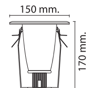
WL-P4016-2KG 130 W150xH170mm E27=1x40W ឧត្តមជ័យ
