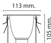
WL-3505B-1KG 90 W113xH105 mm E27=1x40W
