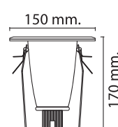
WL-L4015-5YY 130 W150xH170mm E27=1x40W ອລຸມິນຽມ
