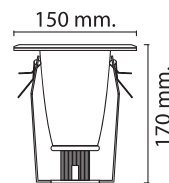
WL-L4015-2YY 130 W150xH170mm E27=1x40W ອລຸມິນຽມ
