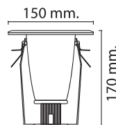
WL-P4016-1KG 130 W150xH170mm E27=1x40W ឧត្តមជ័យ
