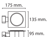
WL-4202-4WH 220 W135xD175xH95 mm E27=1x40W
