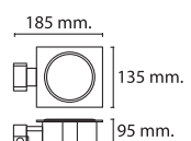
WL-4202-4SN 220 W135xD185xH95 mm E27=1x40W
