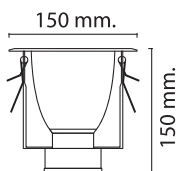
WL4031-A-SS 180 W150xH150 mm E27=1x40W ឧត្តមជ័យ
