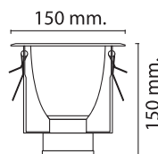
WL-4012A-SN/N 180 W150xH150 mm E27=1x40W ឧត្តមជ័យ
