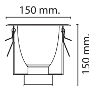
WL4032-A-KG 180 W150xH150 mm E27=1x40W ឧត្តមជ័យ
