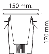
WL-L4015-1YY 130 W150xH170mm E27=1x40W ອລຸມິນຽມ
