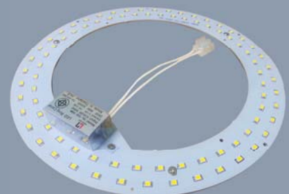
LED-220V-18W 400 แสง 3000K , 6400K ใช้สำหรับชุดเพดาน 32W ต่อตรง ติดตั้งมีแม่เหล็กในตัว
