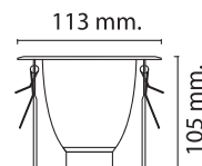
WL-301B-KG 80 W113xH105 mm E27=1x40W
