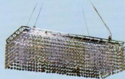
WL-11335-660EL CH-LED 16000 W250xD600xH200 mm E14=10x40W
