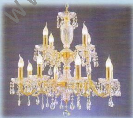
WL-6112-8+4KG 22000 \Phi 710xH650 mm E14=12x40W
