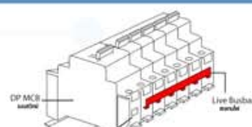
Fixing Busbar การติดตั้งบาร์
